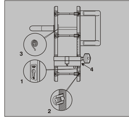
1. Sicherheits-Set Spezialeinlage 2. Stahlkugel 3. Rückholfeder 4. Sicherheitsprofilzylinder
