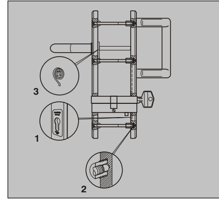
1. Sicherheits-Set Spezialeinlage 2. Stahlkugel 3. Rückholfeder
